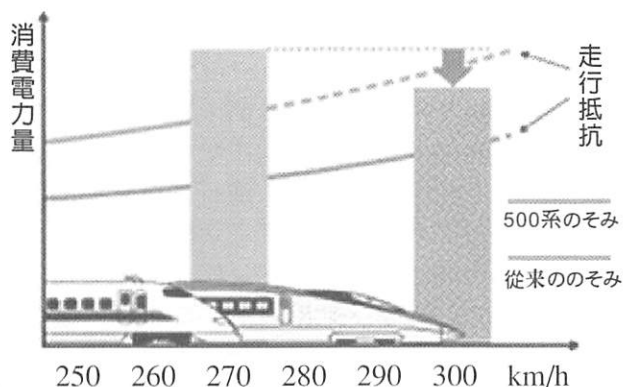
▲ 500 系列電車的電力消耗量 (資料來源 JR 西日本網站)
