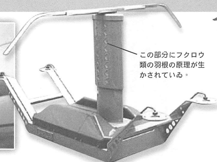
▲ 500 系列電車車頂上之翼型集電装置 (照片提供 JR 西日本)
